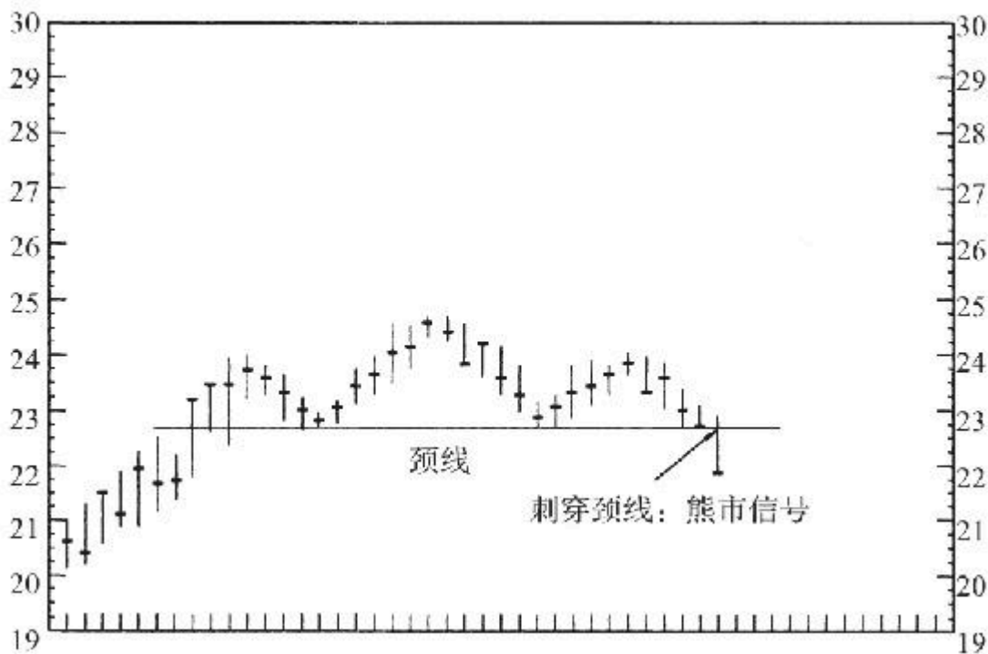
图5-2 头肩顶形态
